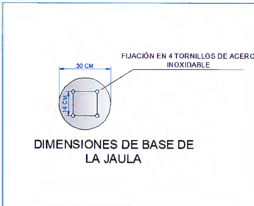
Figura 2. Base de la jaula que alberga linterna en boya.
