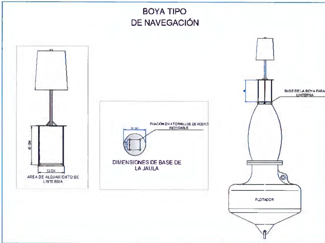
Figura 1. Boya de 1500 mm dm modelo SL-B1500
