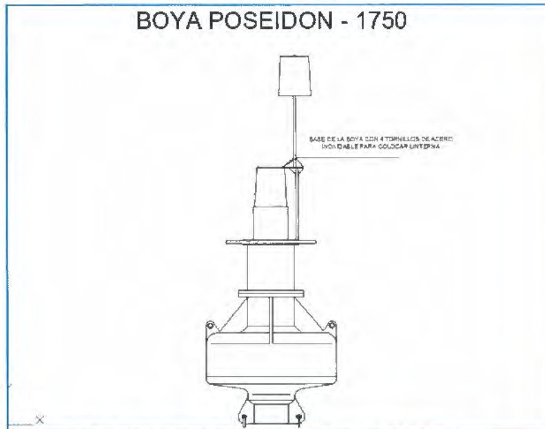
Figura 3. Boya de 1750 mm dm modelo POSEIDON
