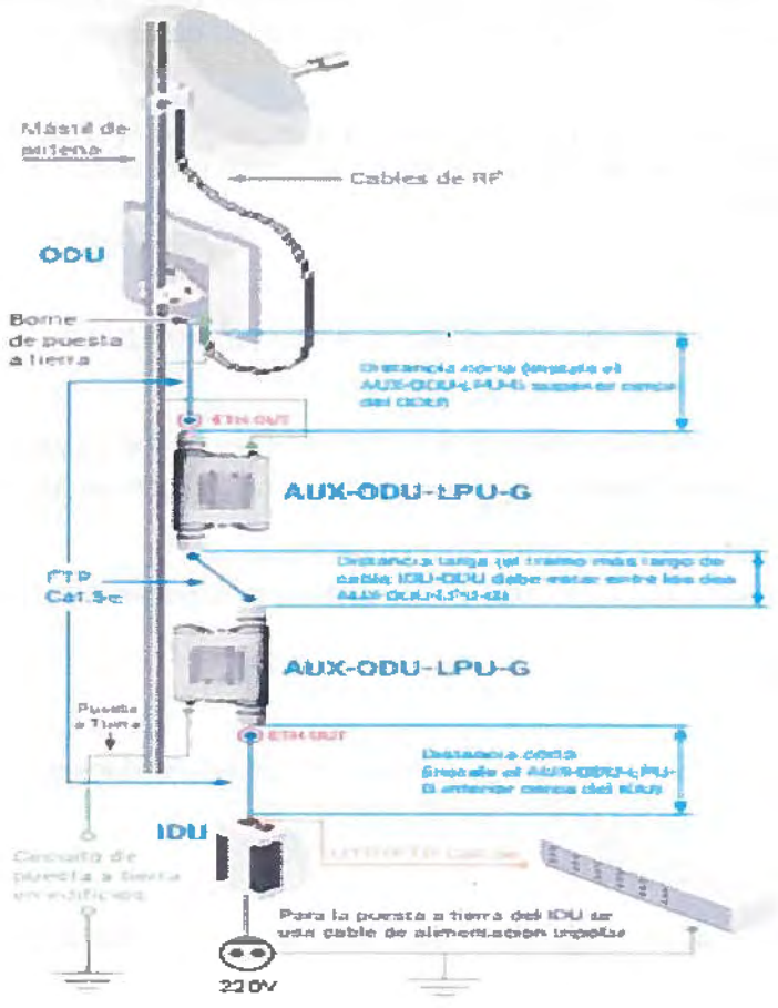
Figura 2. Diagrama Típico de Conexión del enlace.
