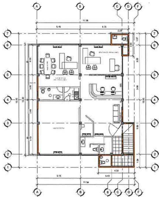
2 Planta alta 1 : 75
