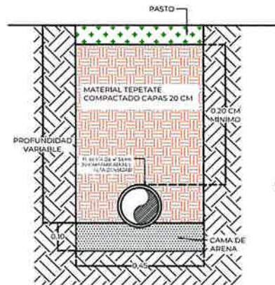
DETALLE DE LINEA DE DRENAJE SANITARIO
