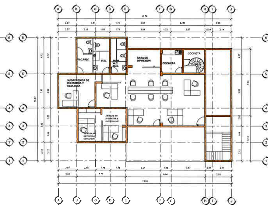
2 Planta General PA 1 : 75
