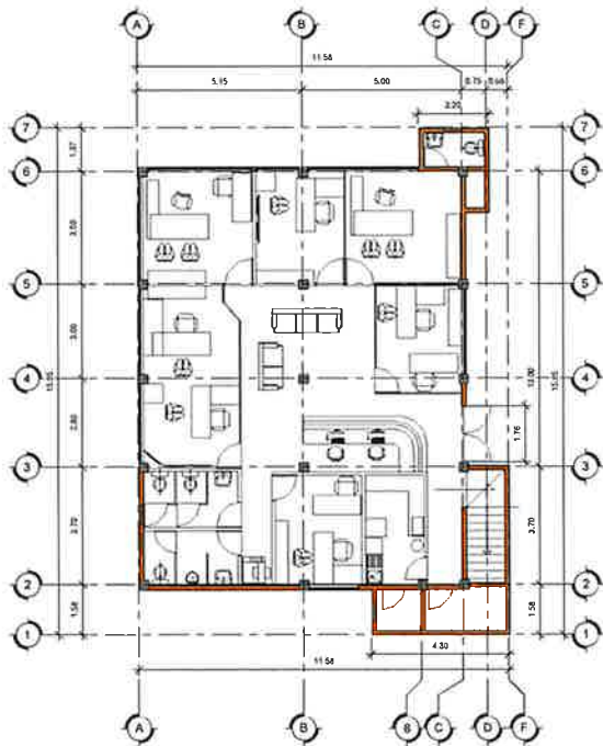
1 Planta Baja 1 : 75
